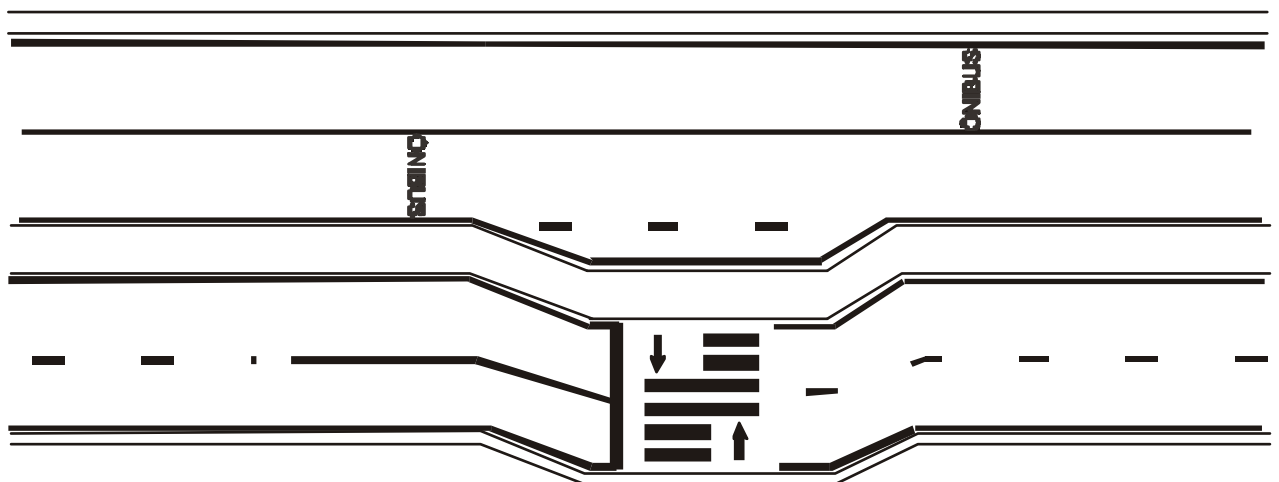
Acesso a ponto de parada de ônibus em pista exclusiva. (recomenda-se a seta na cor branca)
